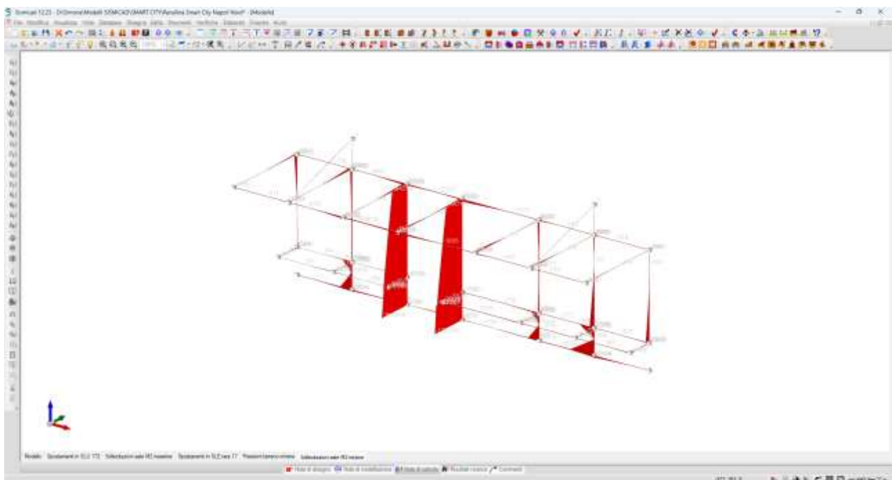
Figura 7. Involuppo momento M2 SLU/SLV
