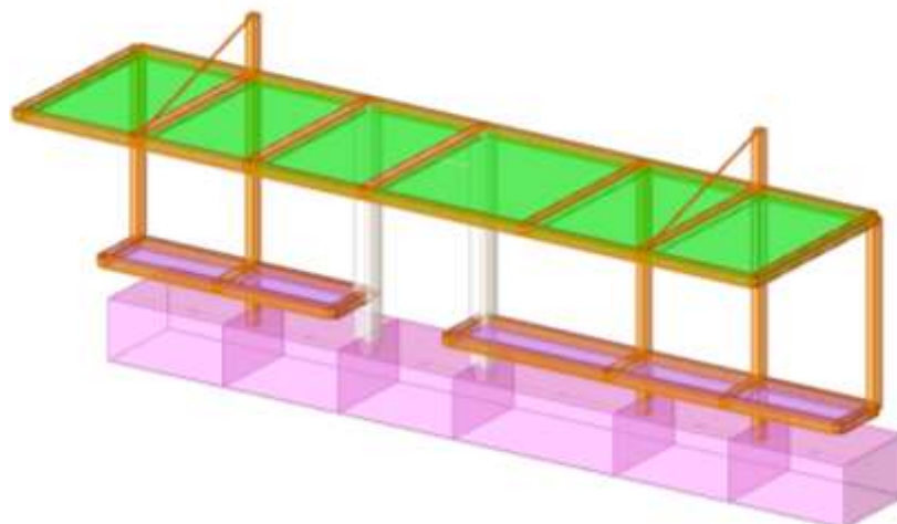
Figura 2. Vista 3D del modello geometrico
